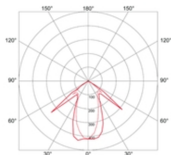
BARI II DLN MH
